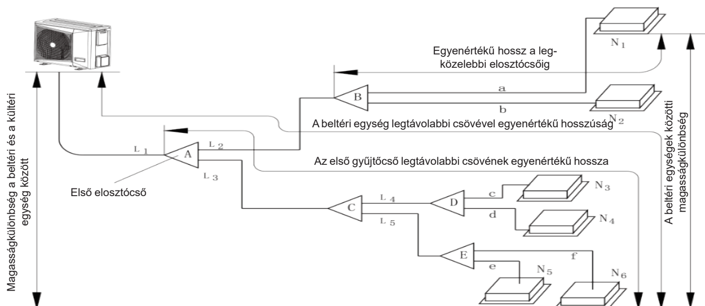
Csatlakozási mód 2
