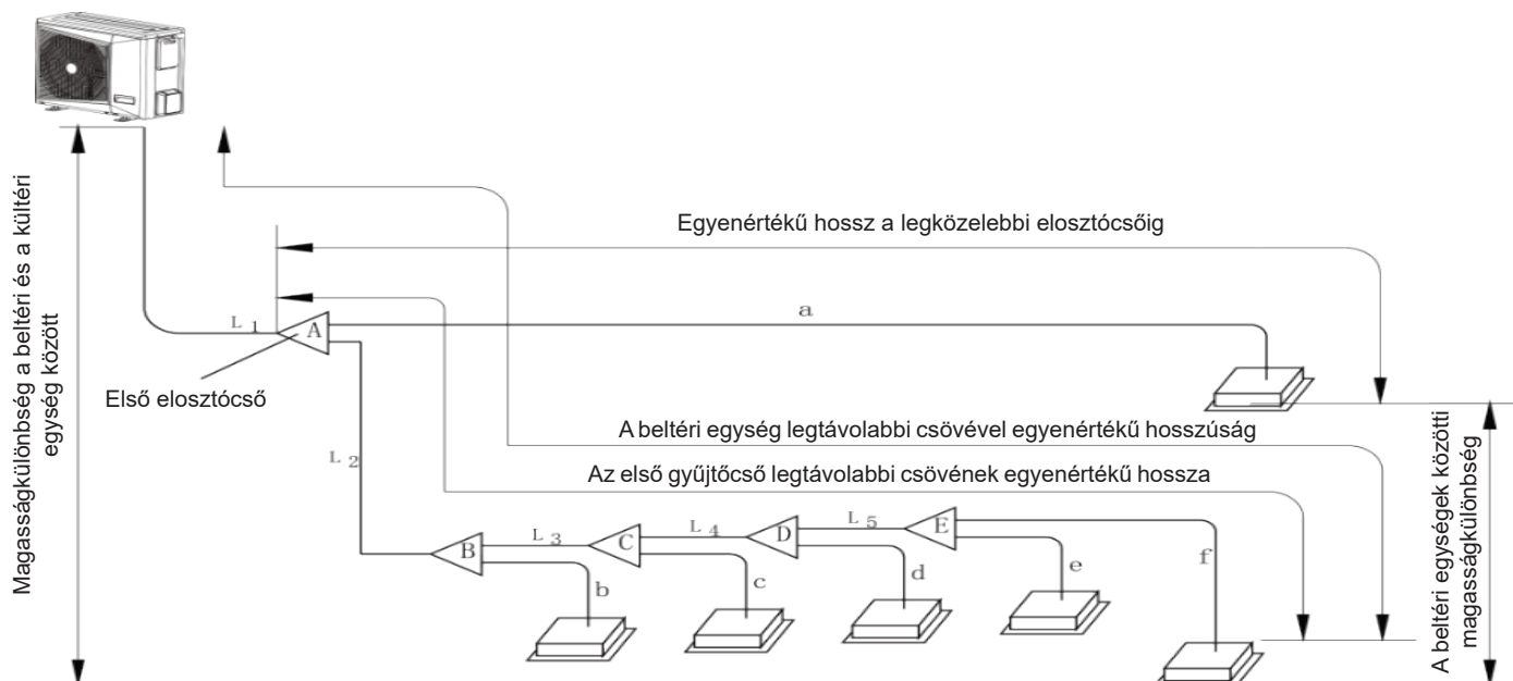
Csatlakozási mód 1
